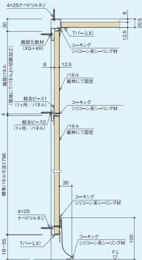
パネル縦断面図(標準パネル仕様)
