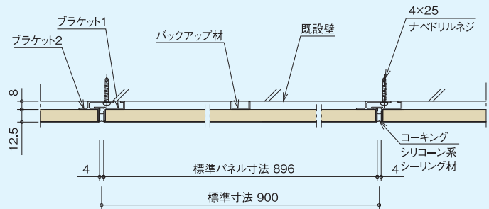
断面：壁
